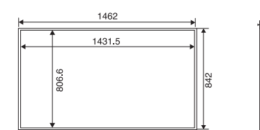
●外形寸法図(単位:mm)
