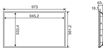
●外形寸法図(単位:mm)
