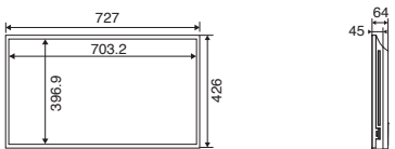
●外形寸法図(単位:mm)
