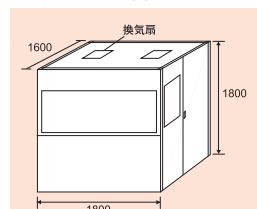
●通訳ブース寸法図 (単位:mm)
