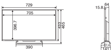
●外形寸法図(単位:mm)
