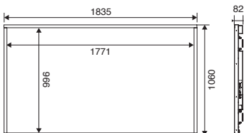
●外形寸法図(単位:mm)
