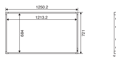
●外形寸法図(単位:mm)
