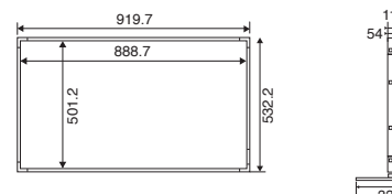
●外形寸法図(単位:mm)
