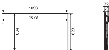
●外形寸法図(単位:mm)
