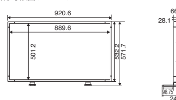
●外形寸法図(単位:mm)
