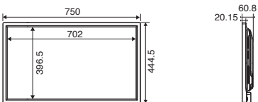
●外形寸法図(単位:mm)
