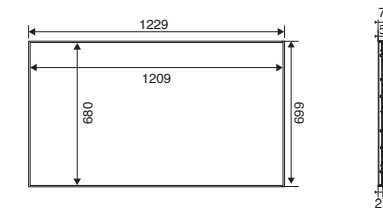
●外形寸法図(単位:mm)
