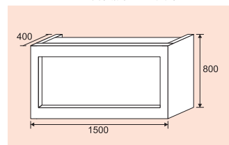
●パーテーション寸法図(会議机の上に設置)(単位:mm)
