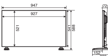
●外形寸法図(単位:mm)
